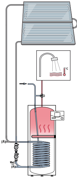
Solarni sistem bez ekspanzione posude
